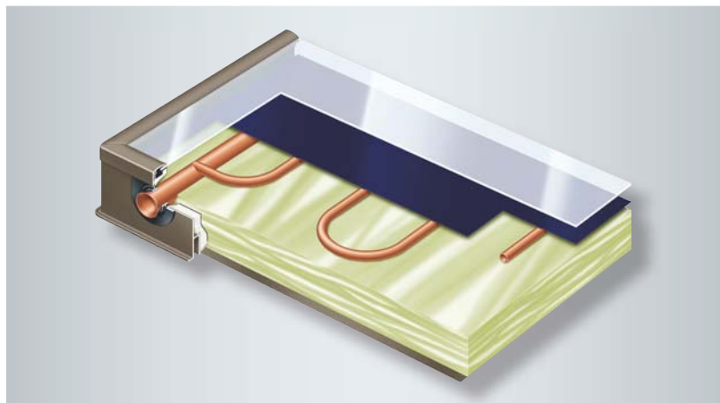
Vitosol 200-F mit Sol-Titan-Beschichtung
