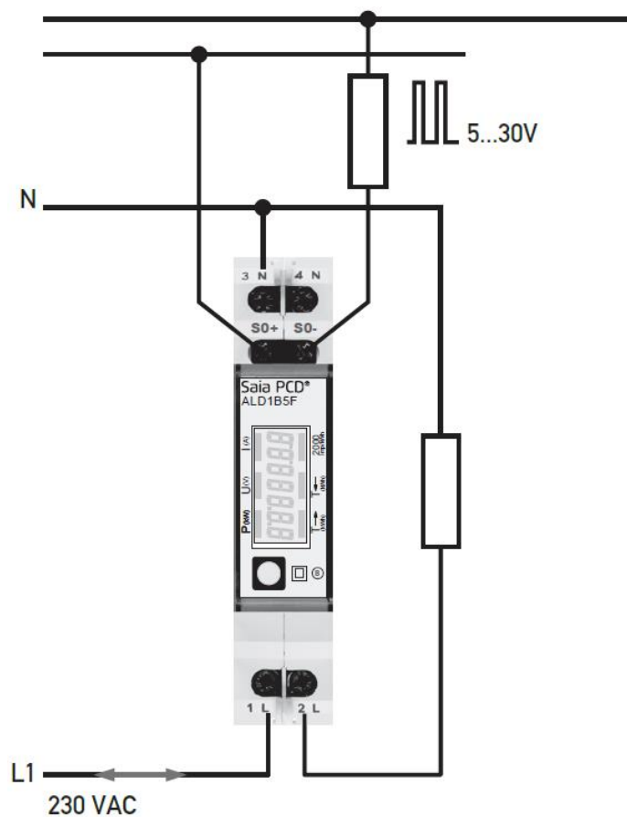
Abbildung 4 – Anschlussbild
