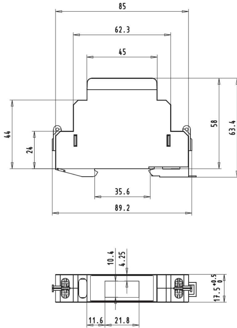
Abbildung 5 - Zählergehäuse
